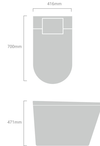
慕尼黑尺寸图 Munich's dimensions
