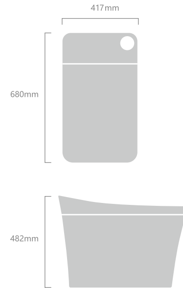
汉诺威尺寸图 Hannover's dimensions
